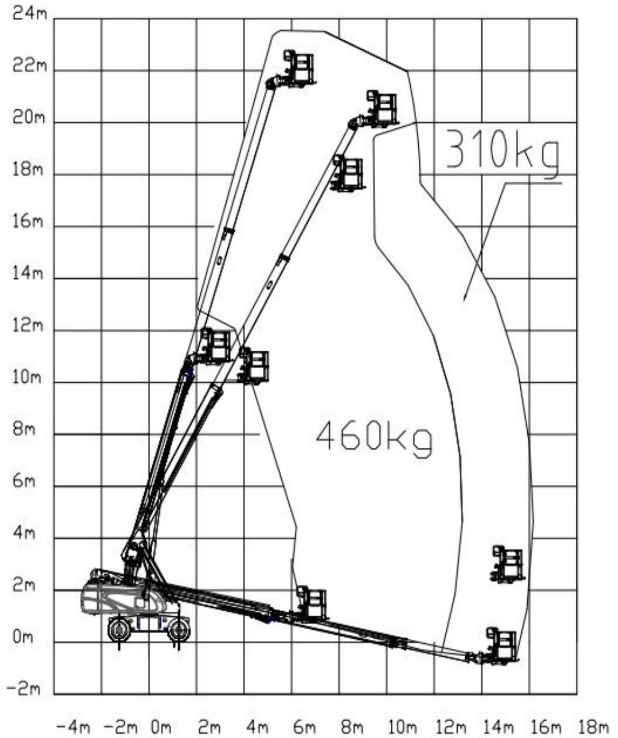
图 1-3 HB230P 作业范围图
