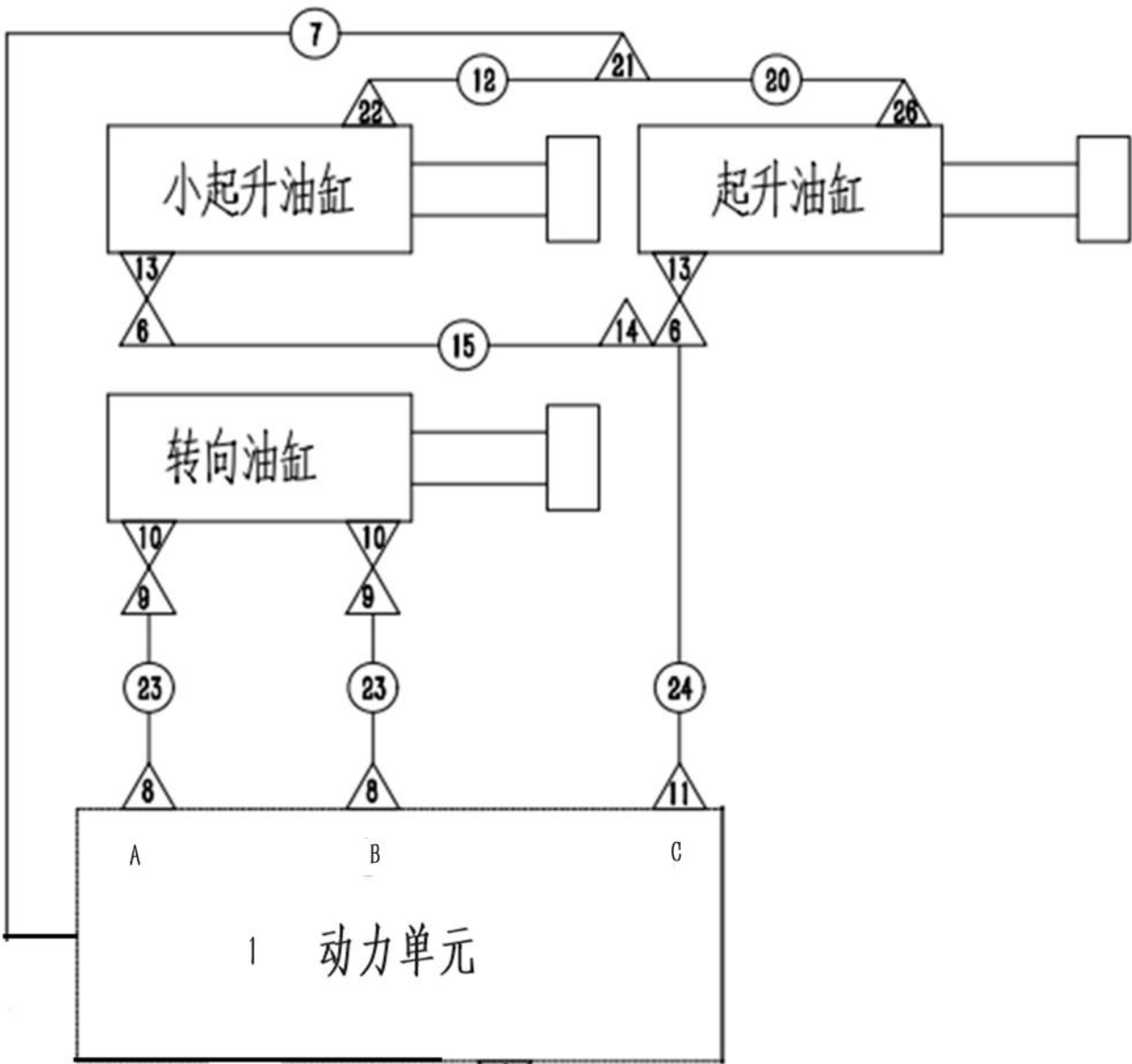
4-1 胶管连接示意图
