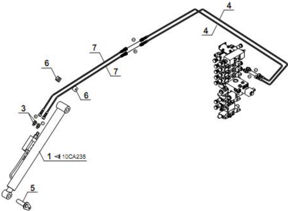
图 5-6 液压油路-摆臂油路（GTHZ120）
