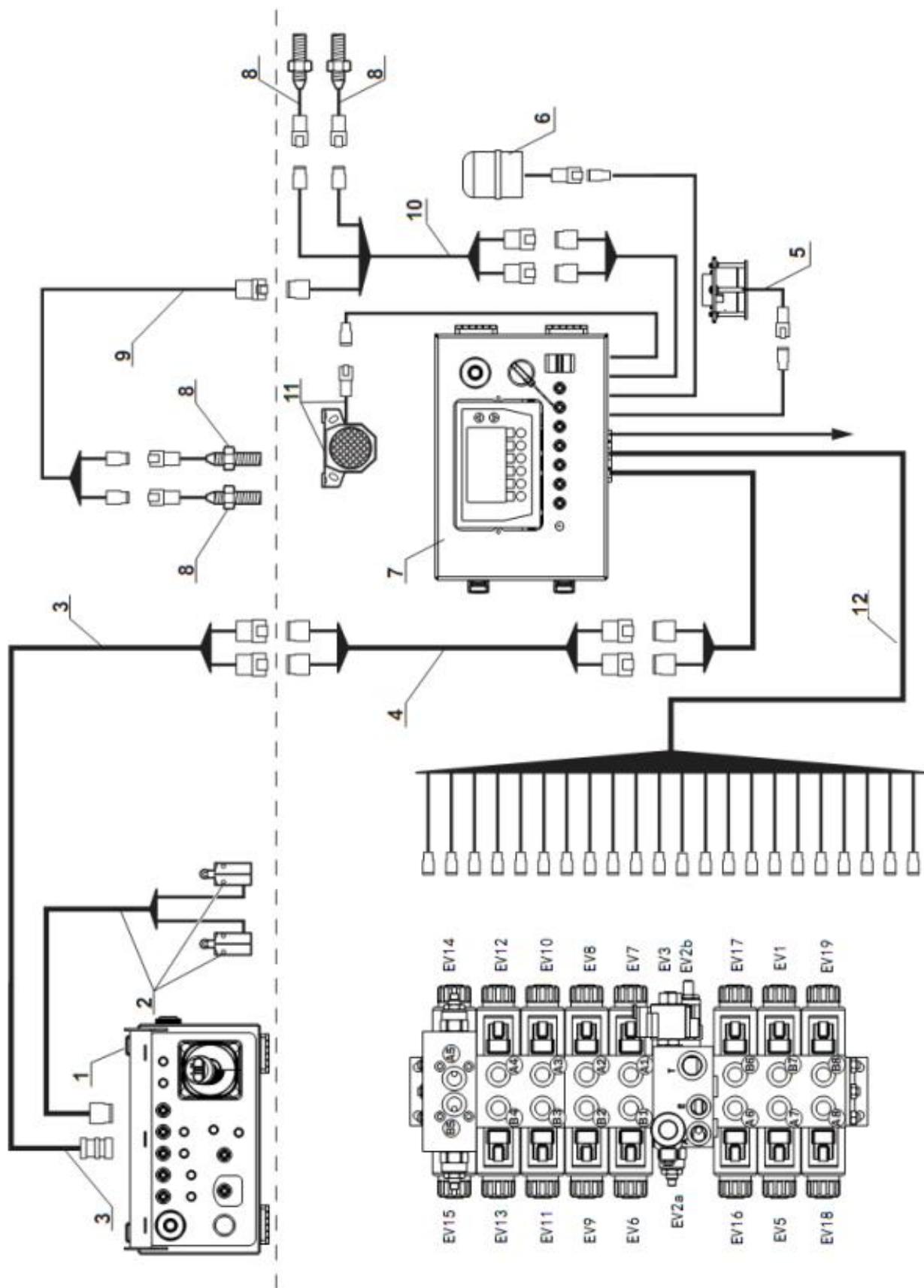
图 6-2 接线图一（GTHZ170/GTHZ170C）
