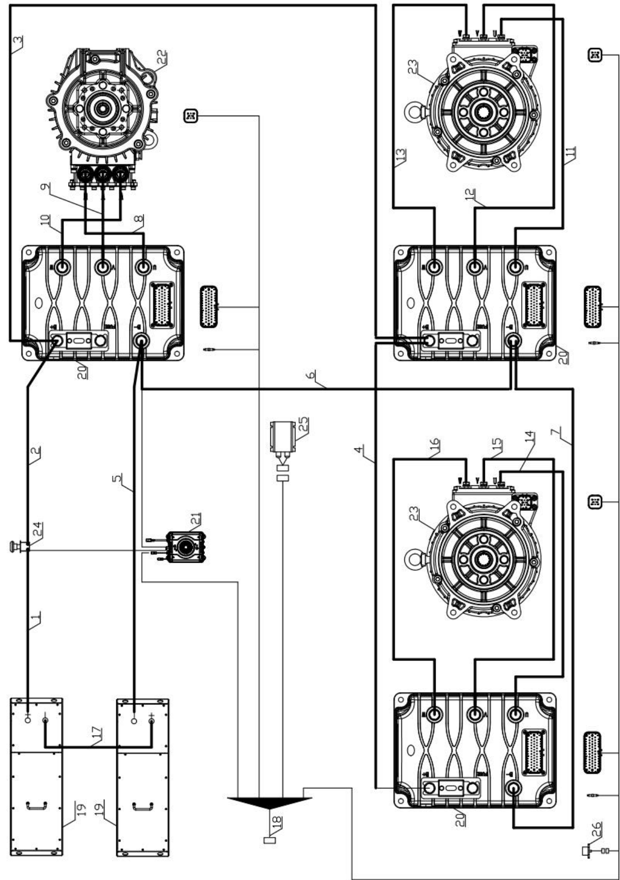
图 6-3 接线图二（铅酸电池）
