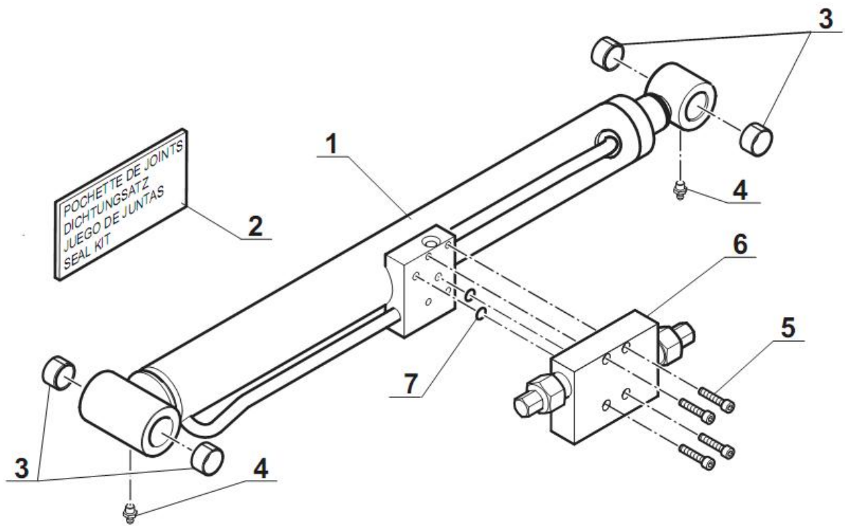
图 5-23 摆臂油缸组件
