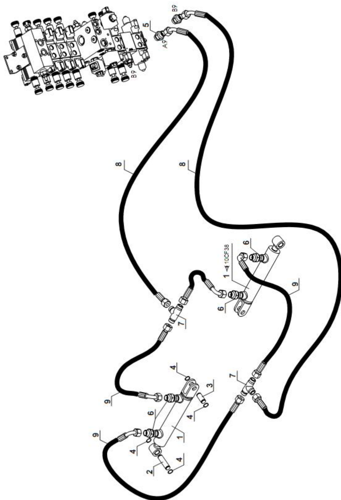
图 5-15 液压油路-防倾翻油路 (GTHZ120)
