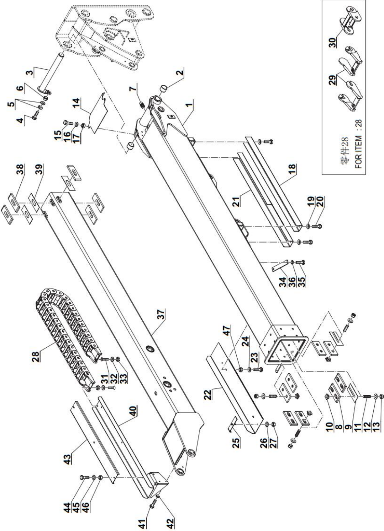
图 3-3 上臂与伸缩臂装配 (GTHZ120)
