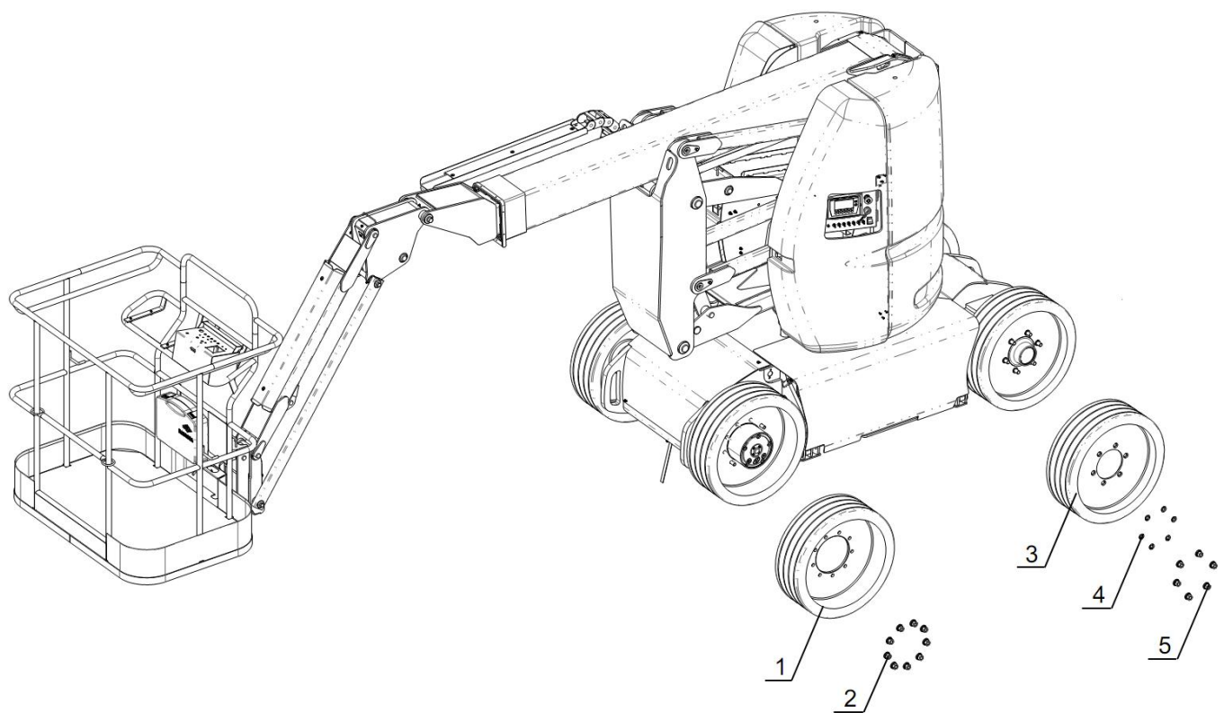
图 1-1 轮胎（GTHZ120）
