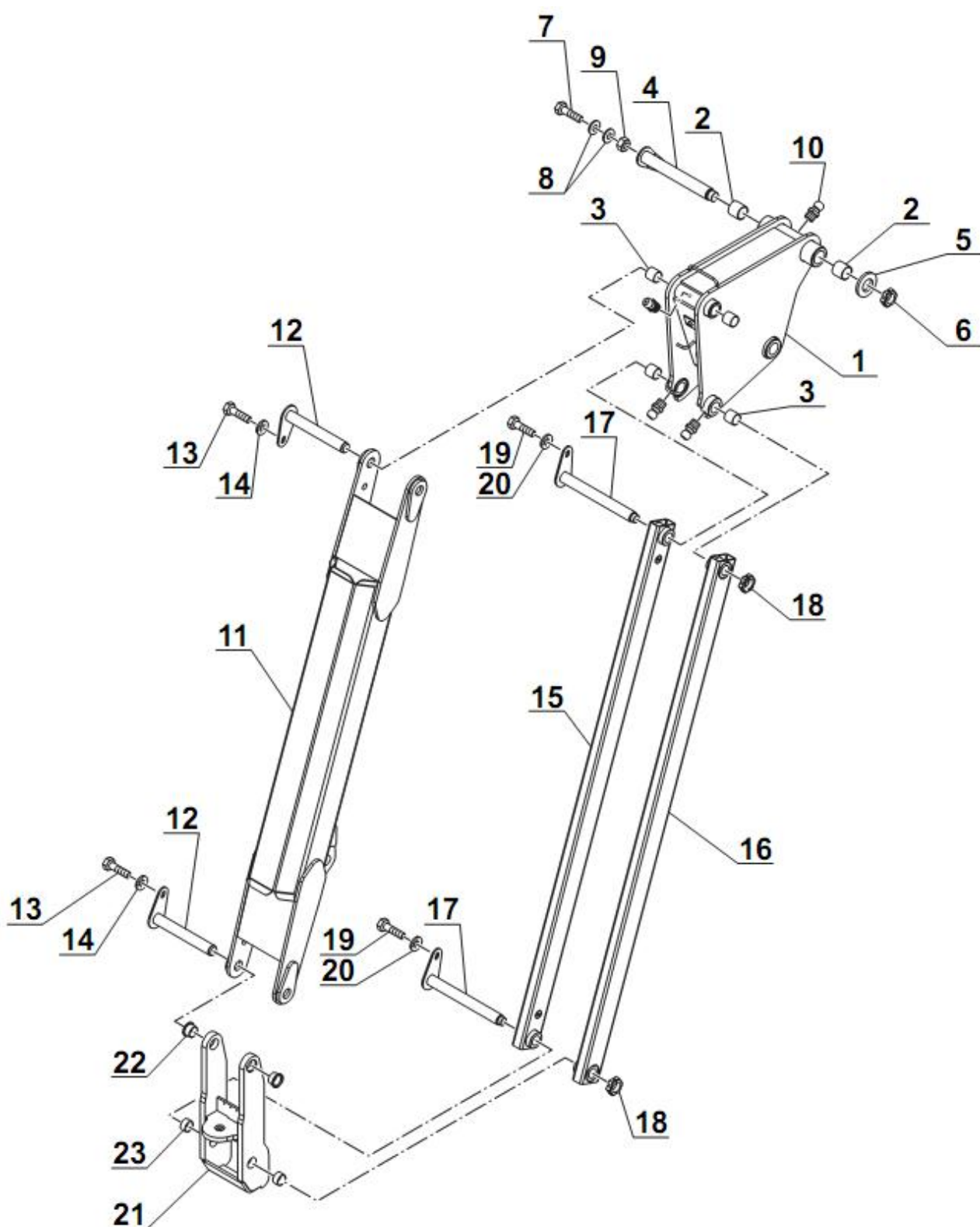
图 3-5 摆臂组件
