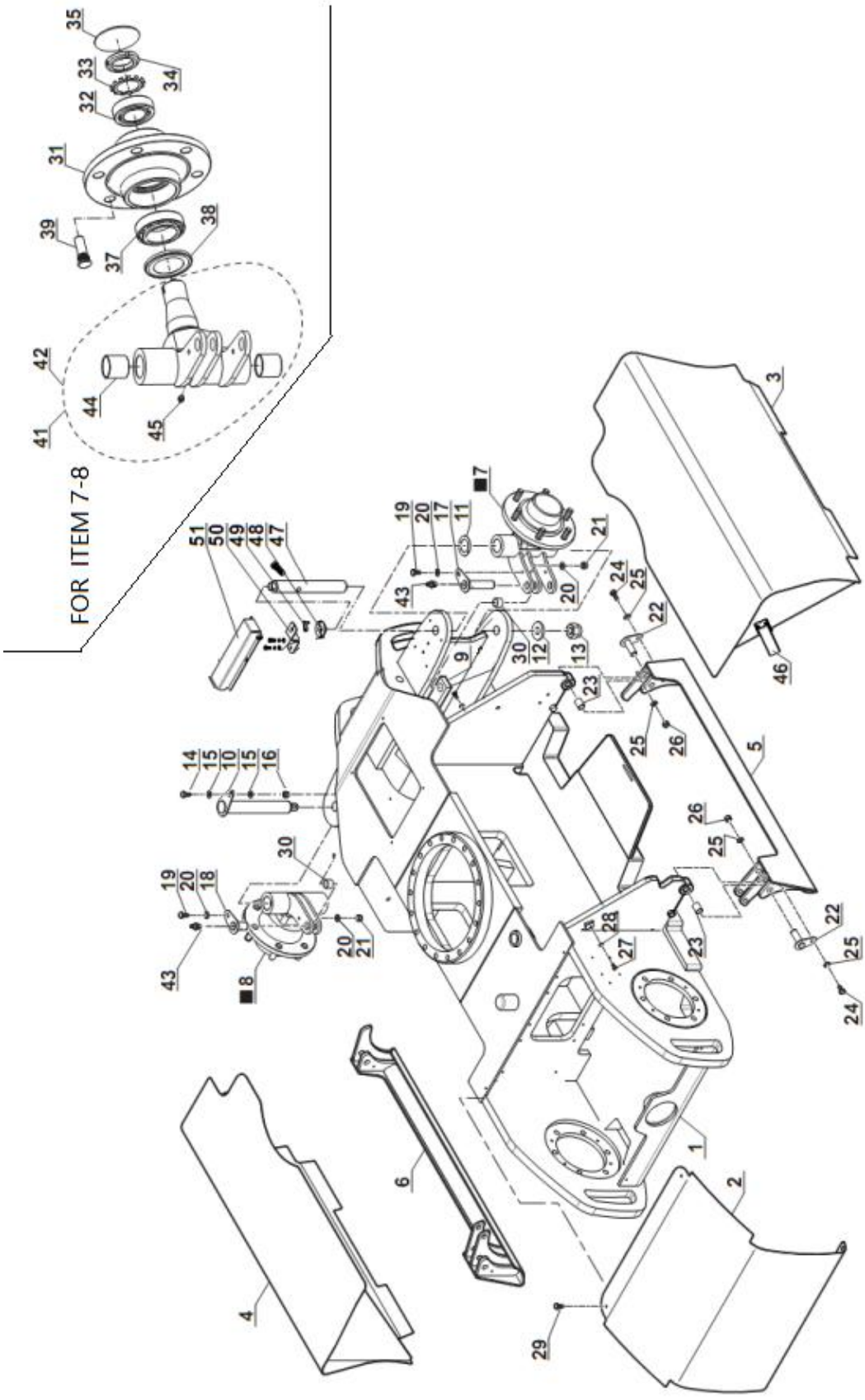
图 1-4 底盘装配 (GTHZ120)
