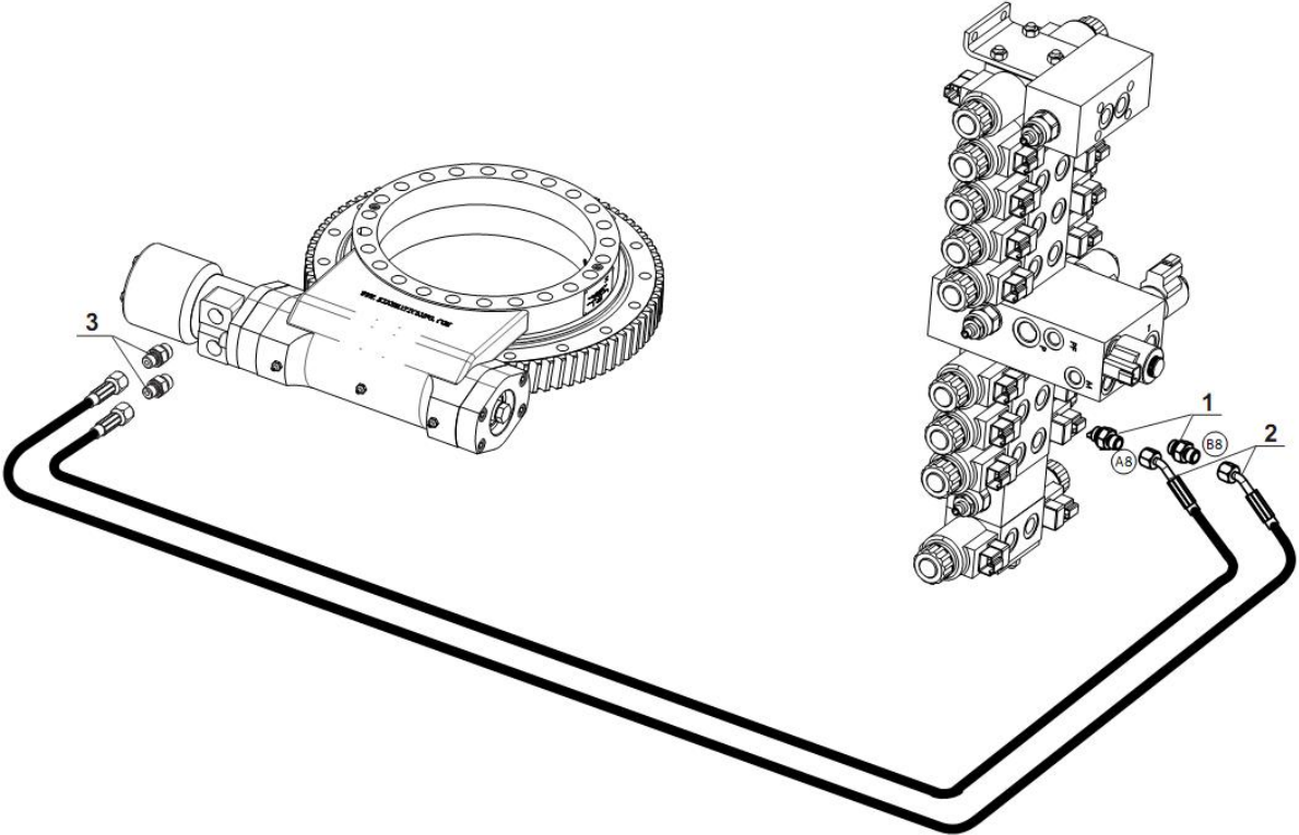
图 5-3 液压油路-塔身旋转油路
