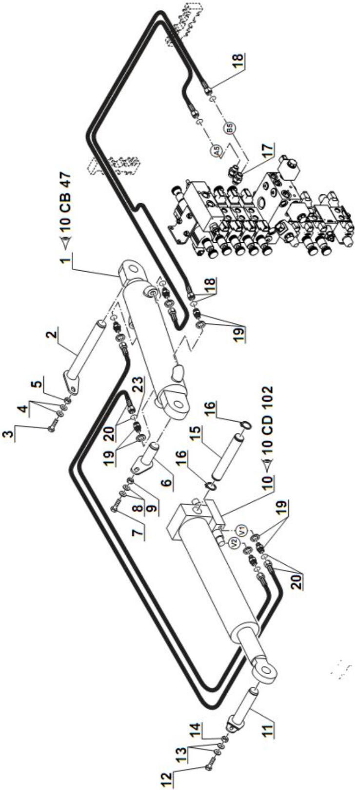
图 5-11 液压油路-调平油路 (GTHZ170/GTHZ170C)
