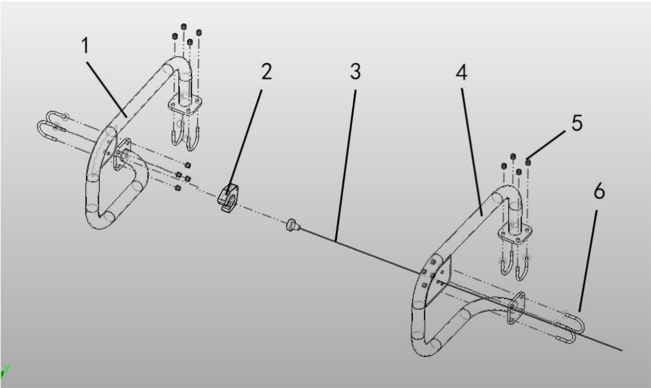
图 4-2 防挤压装置
