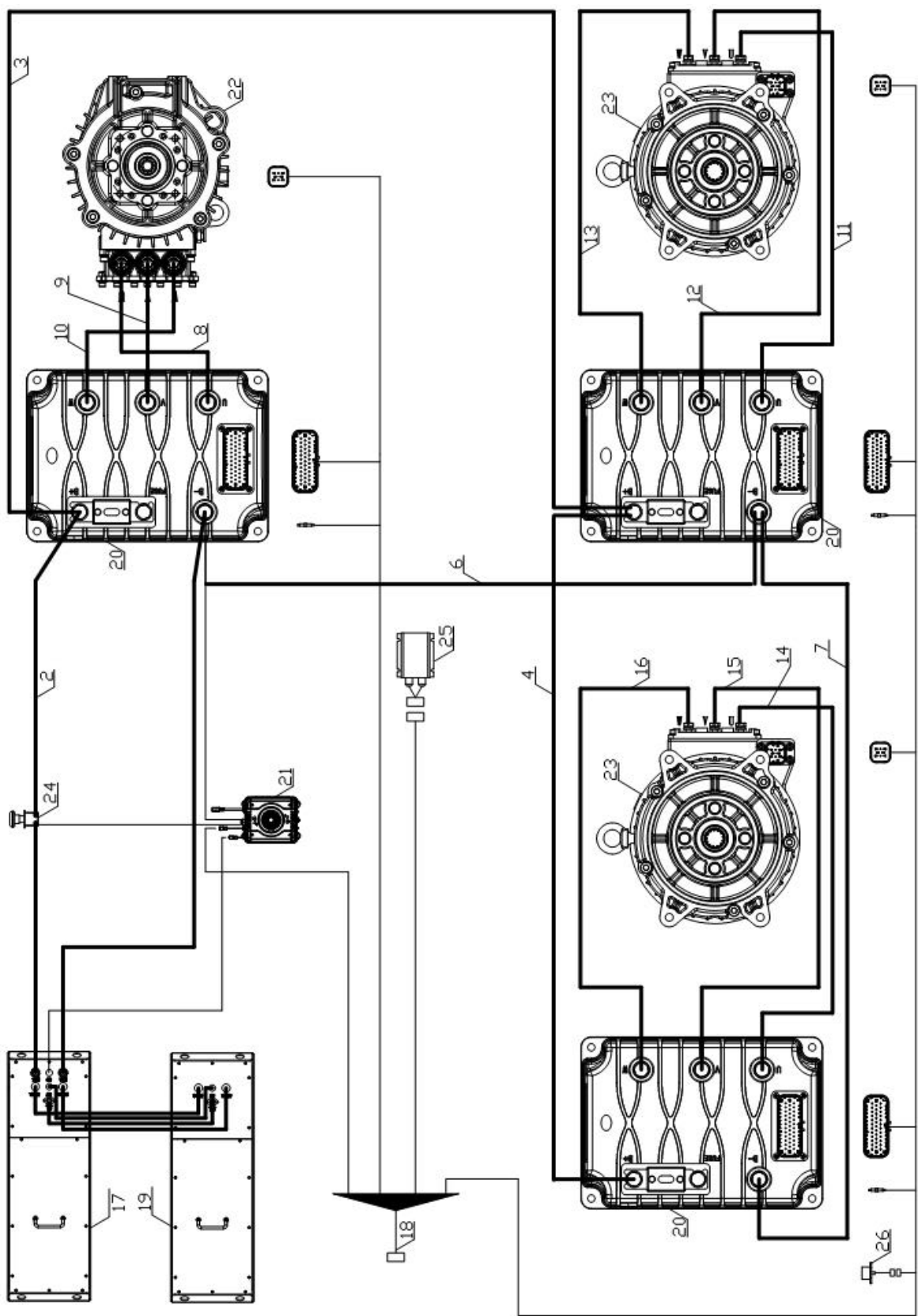
图 6-4 接线图二（锂电池）
