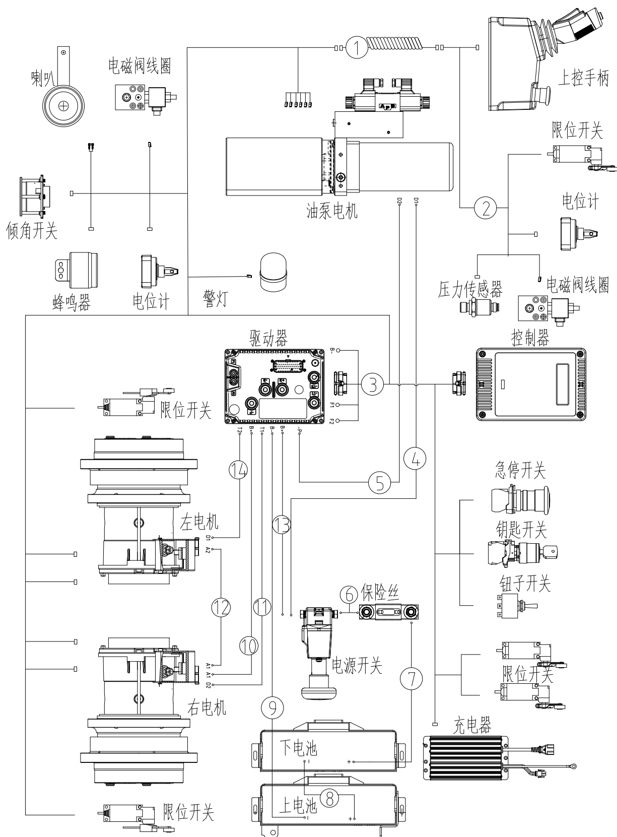
6-1 电气线束
