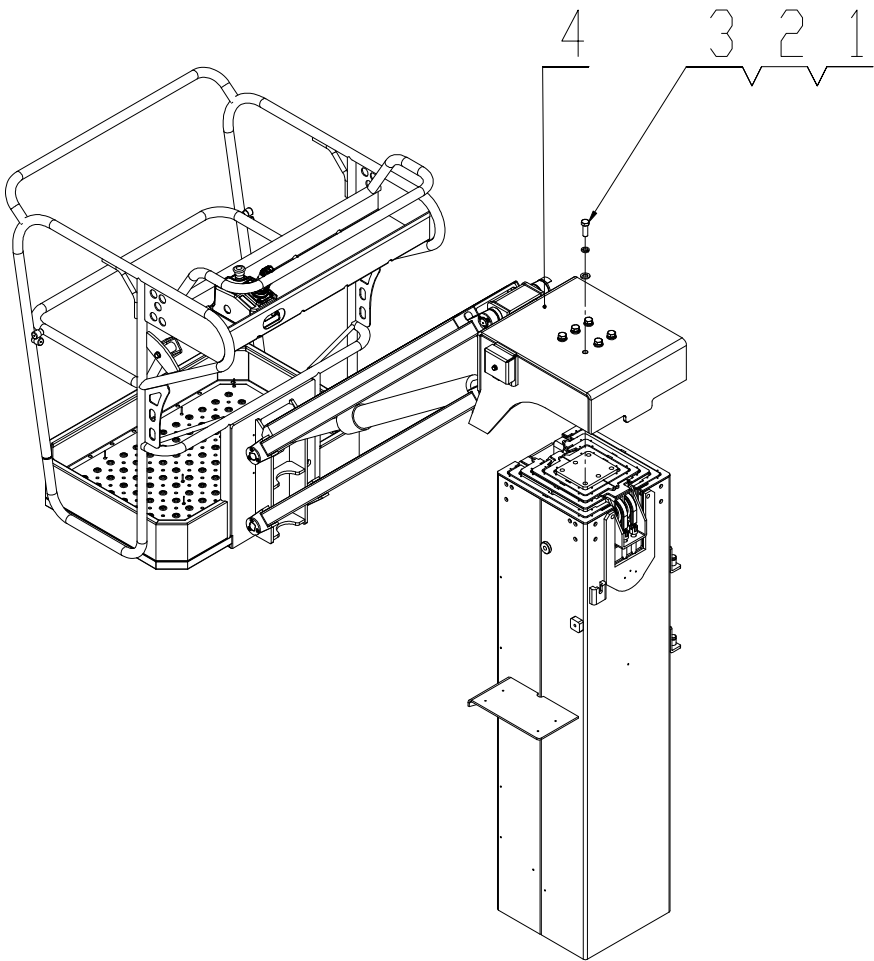
4-1 平台与套管装配
